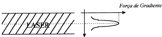
Gráfico 2: Curva (Gaussiana) da intensidade da força de gradiente X região do LASER.
